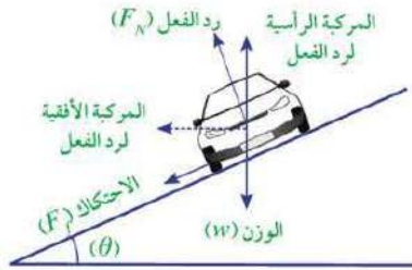
شكل (٩): القوة الجاذبة المركزية هي مجموع مركبتى رد الفعل والاحتكاك في الاتجاه الأفقى
