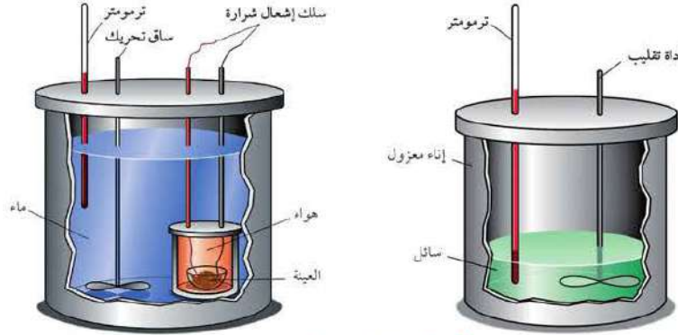
شكل (٣) المسعر الحراري
