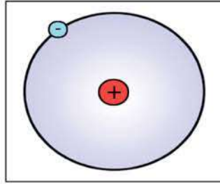
شكل (١٩) قطر الذرة الواحدة
