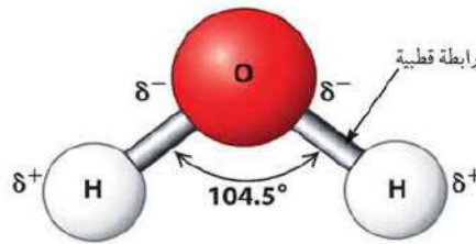
▲ شكل (٤) الزاوية بين الرابطتين في جزيء الماء
