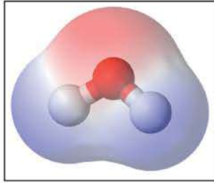
شكل (١٨) لجزيء الماء
