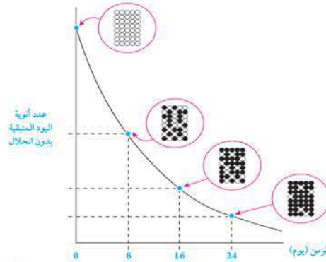
▲ شكل (٨) منحنى انحلال اليود - 131 ، عمر النصف له 8 أيام
